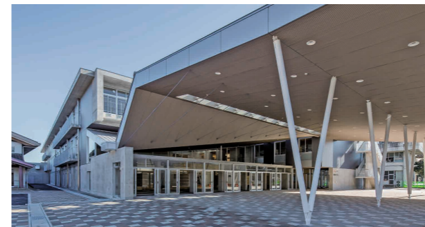
完成した3階建ての新校舎
