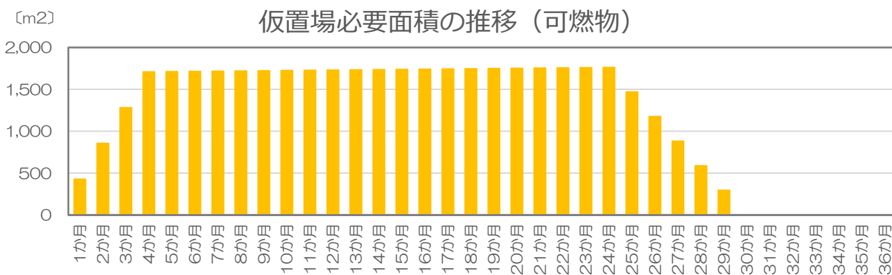
図表 62 月別の仮置場の必要面積の推移（可燃物）
