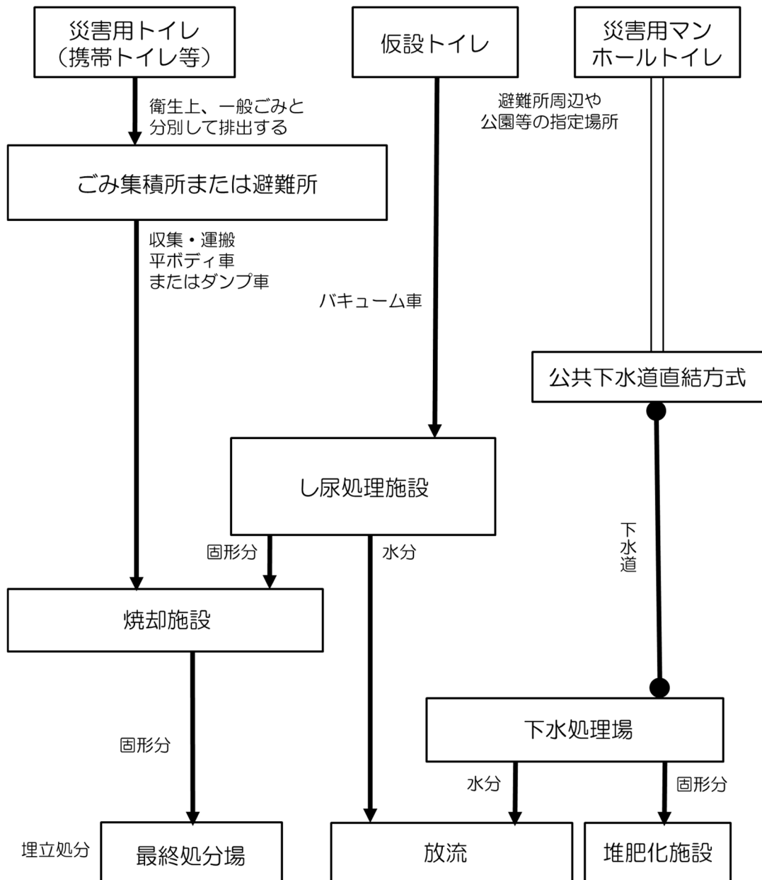
図表 13 し尿処理の流れ
