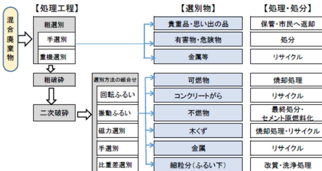
図表 混合廃棄物の処理（例）
