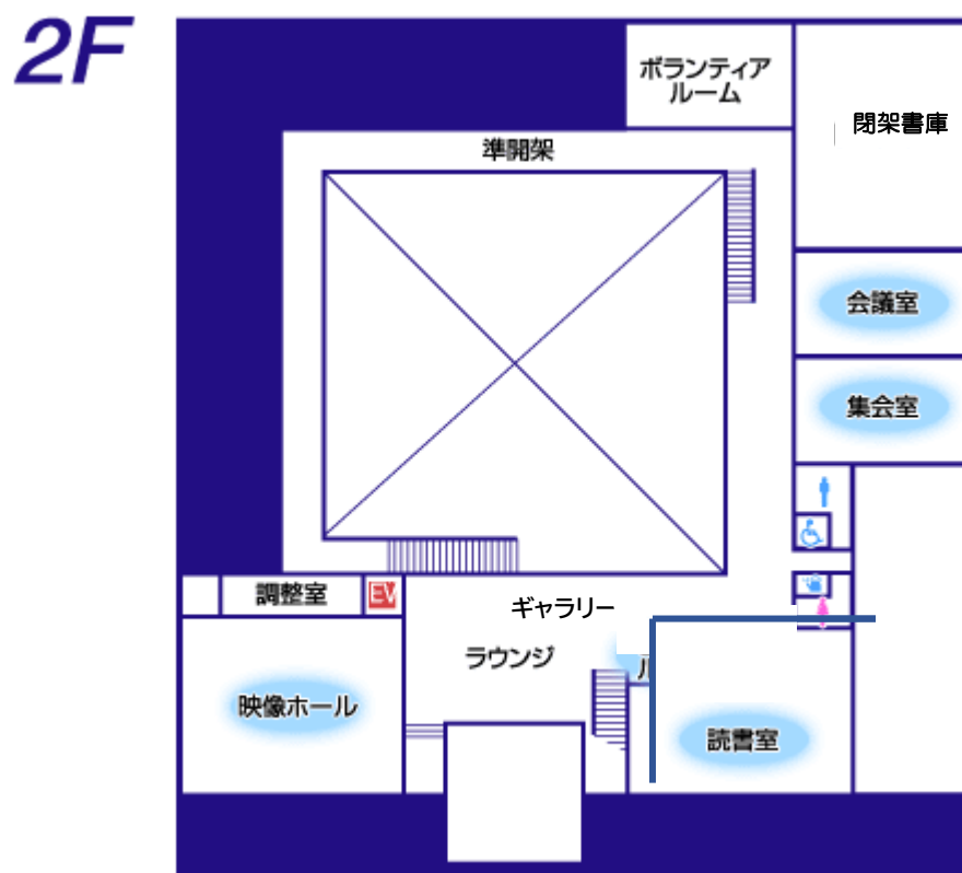
2 階平面図
