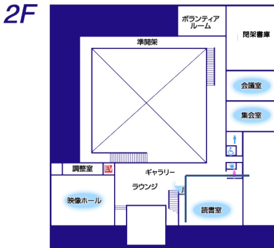
2 階平面図
